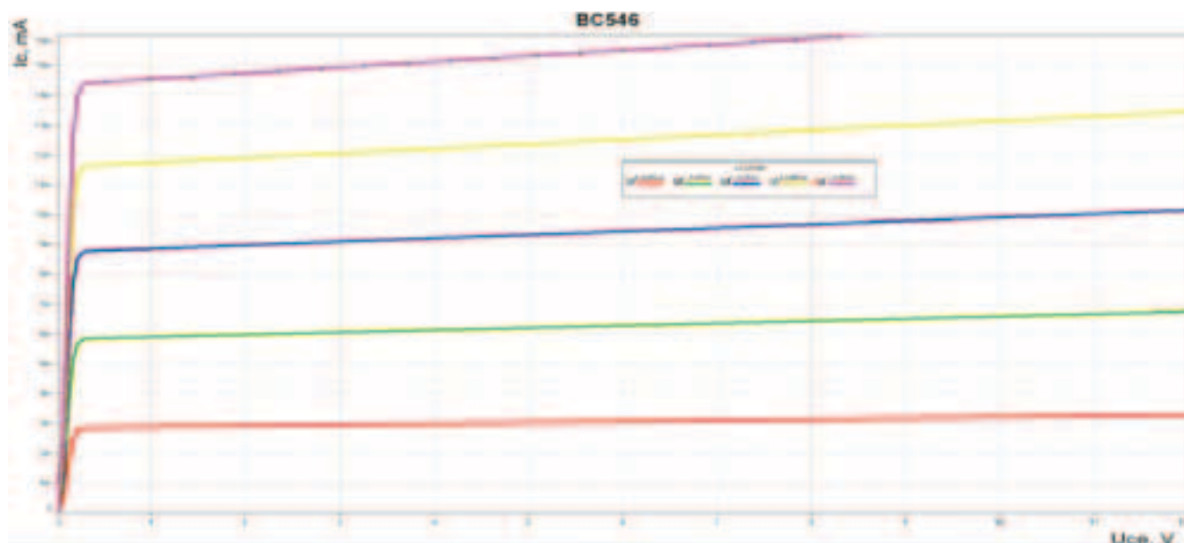
Příloha k příkladu: Výstupní charakteristiky tranzistoru BC546
